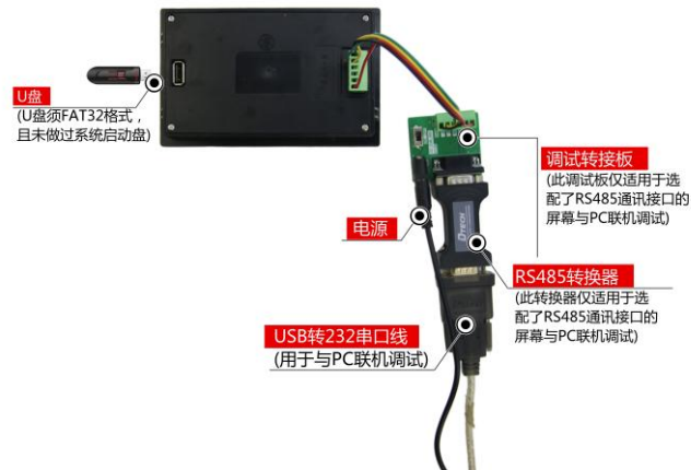
图 1-4 RS485 调试工具图
