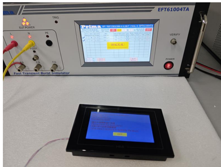
图 5-3 EFT 测试图
