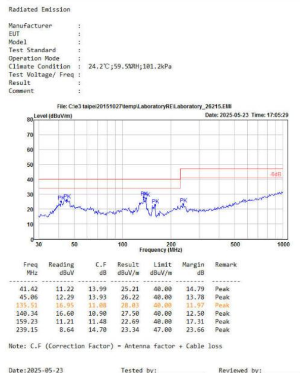
图 5-6 RE 测试垂直方向
